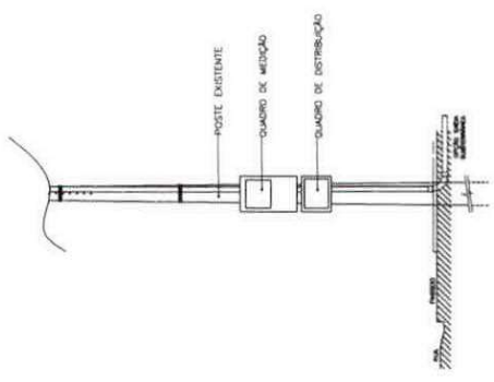
DETALHE MEDIÇÃO "POSTE"
